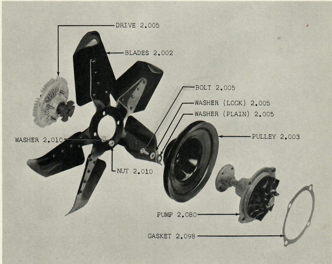
GROUP 2 - FIG. 3 - AUTOMATIC FAN DRIVE 80 (WAF)
